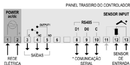
Fig. 01 – Conexões mostradas na etiqueta do controlador
